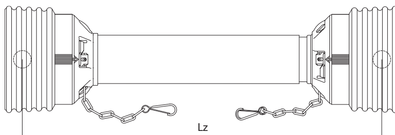
Расстояние (Lz) между центрами крестовин в сложенном виде
