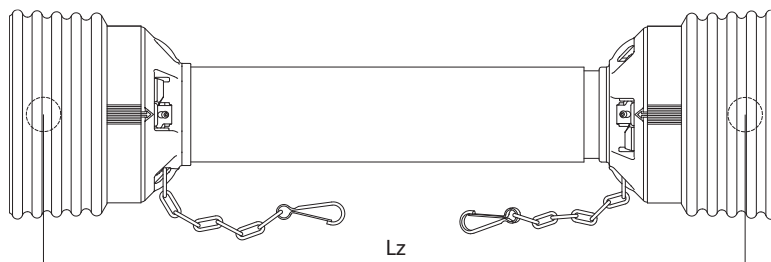
Расстояние (Lz) между центрами крестовин в сложенном виде
