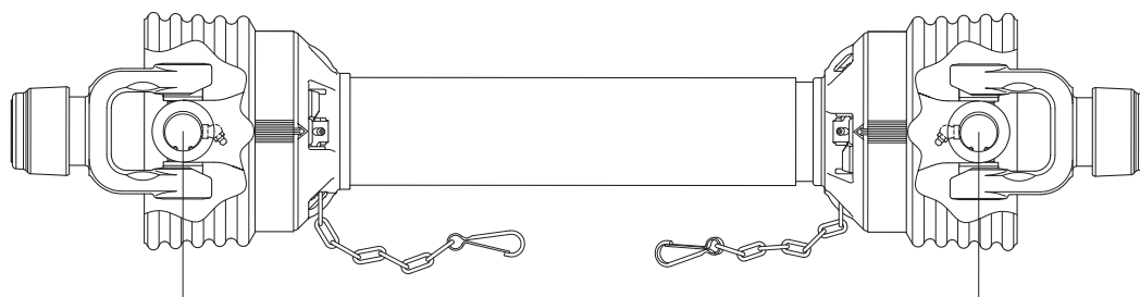
Расстояние (Lz) между центрами крестовин в сложенном виде
