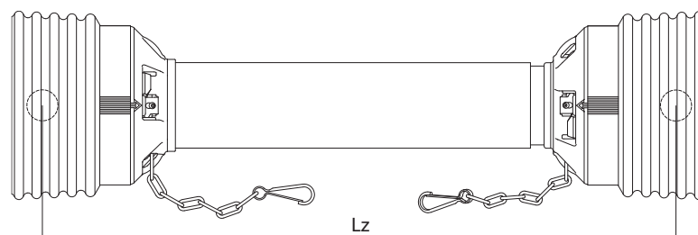
Расстояние между центрами крестовин (Lz) в сложенном виде
